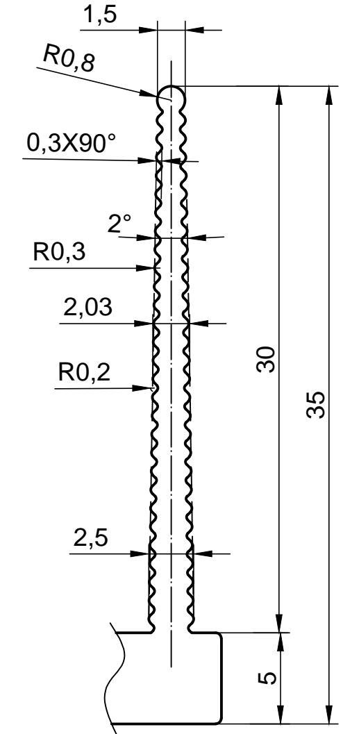
DETAY-A ÖLÇEK 2.5/1
