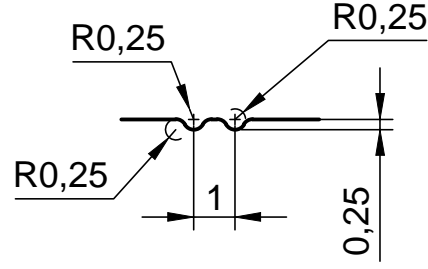
DETAY A ÖLÇEK 4/1
