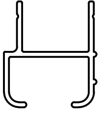
ÖLÇEK 1/1
